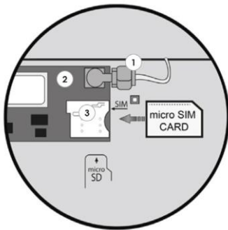
4G/LTE add-on module KSI4104001.300
